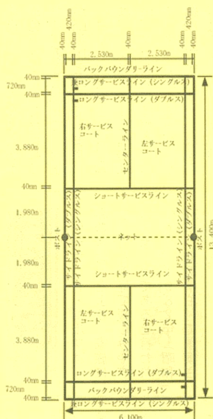
対角線の長さ ダブルス 14.723m シングル 14.366m
