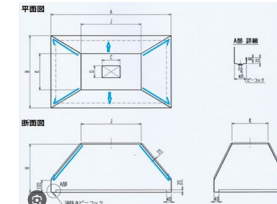
排気用フード設備※参考資料
