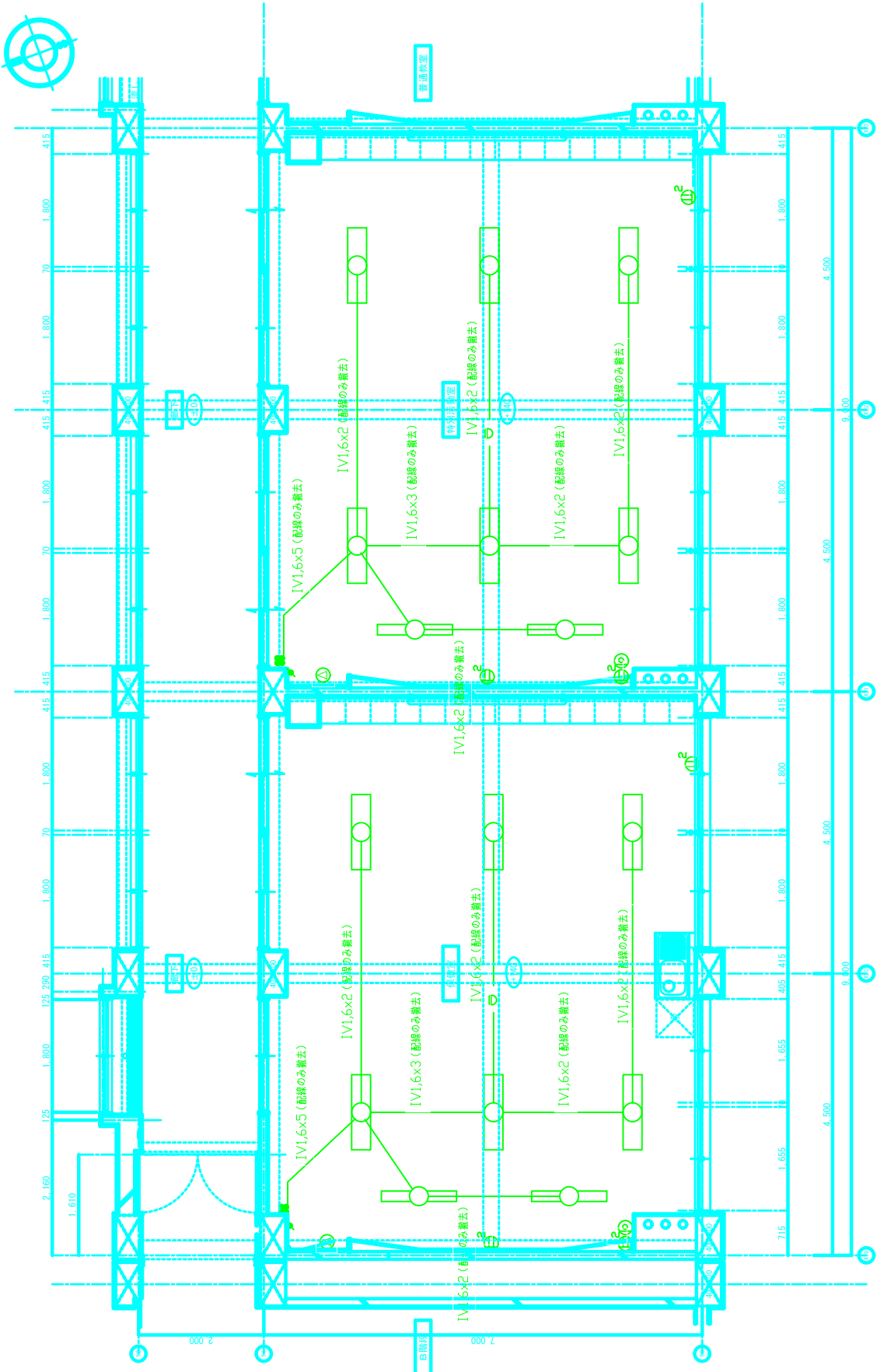
(新)会議室・特別支援教室 平面詳細図(改修) S1:50
